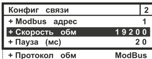
Рисунок 3.26 – Стартовое изображение меню Конфигурация связи
