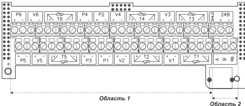
Рисунок Б.1 – Плата подключений вычислителя KARAT-308
